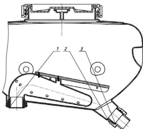
1 Склоп за цевката за прскање 2 Конектор 3 Заптивна подложка
