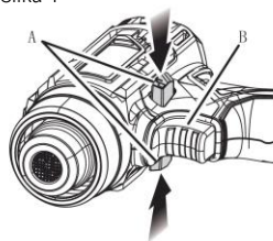
A - Blokirni gumb B - Stikalo za vklop/izklop
